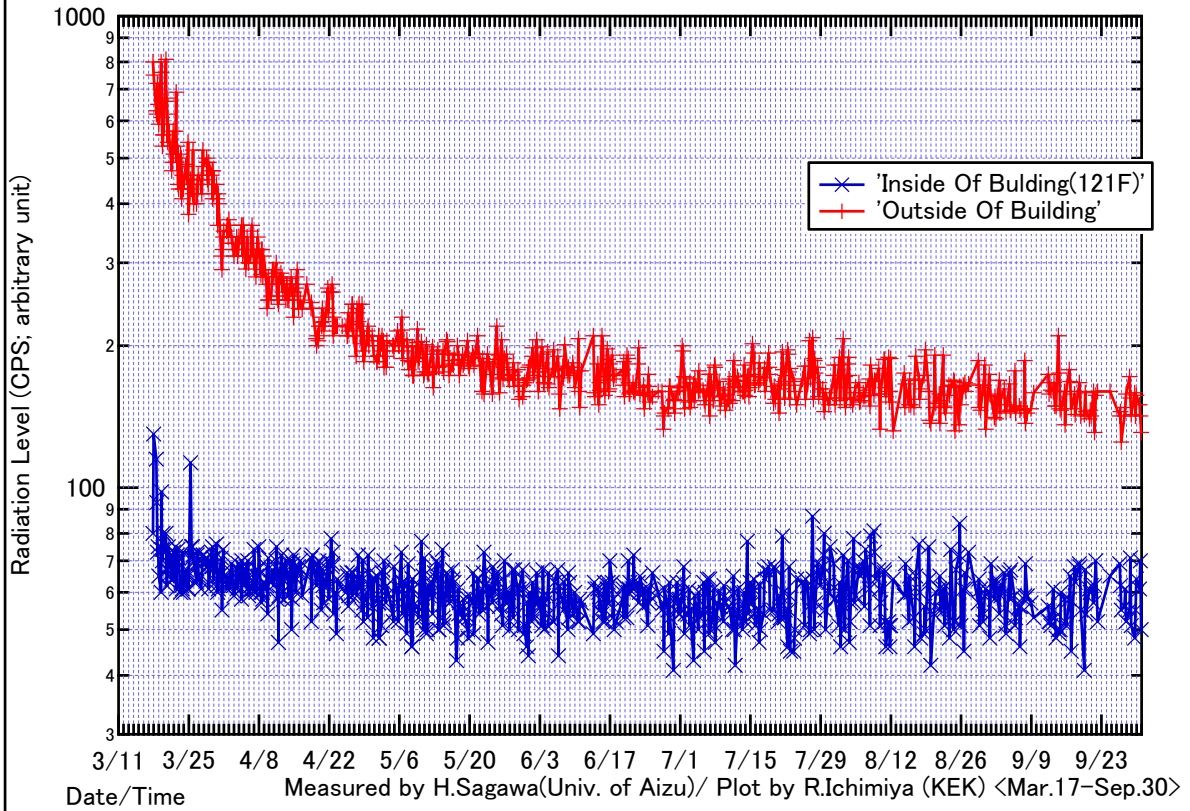
会津大学(福島県会津若松市)環境放射線レベル測定 (GM) Environmental Radiation Level at Univ. of Aizu (Aizuwakamatsu, Fukushima)
