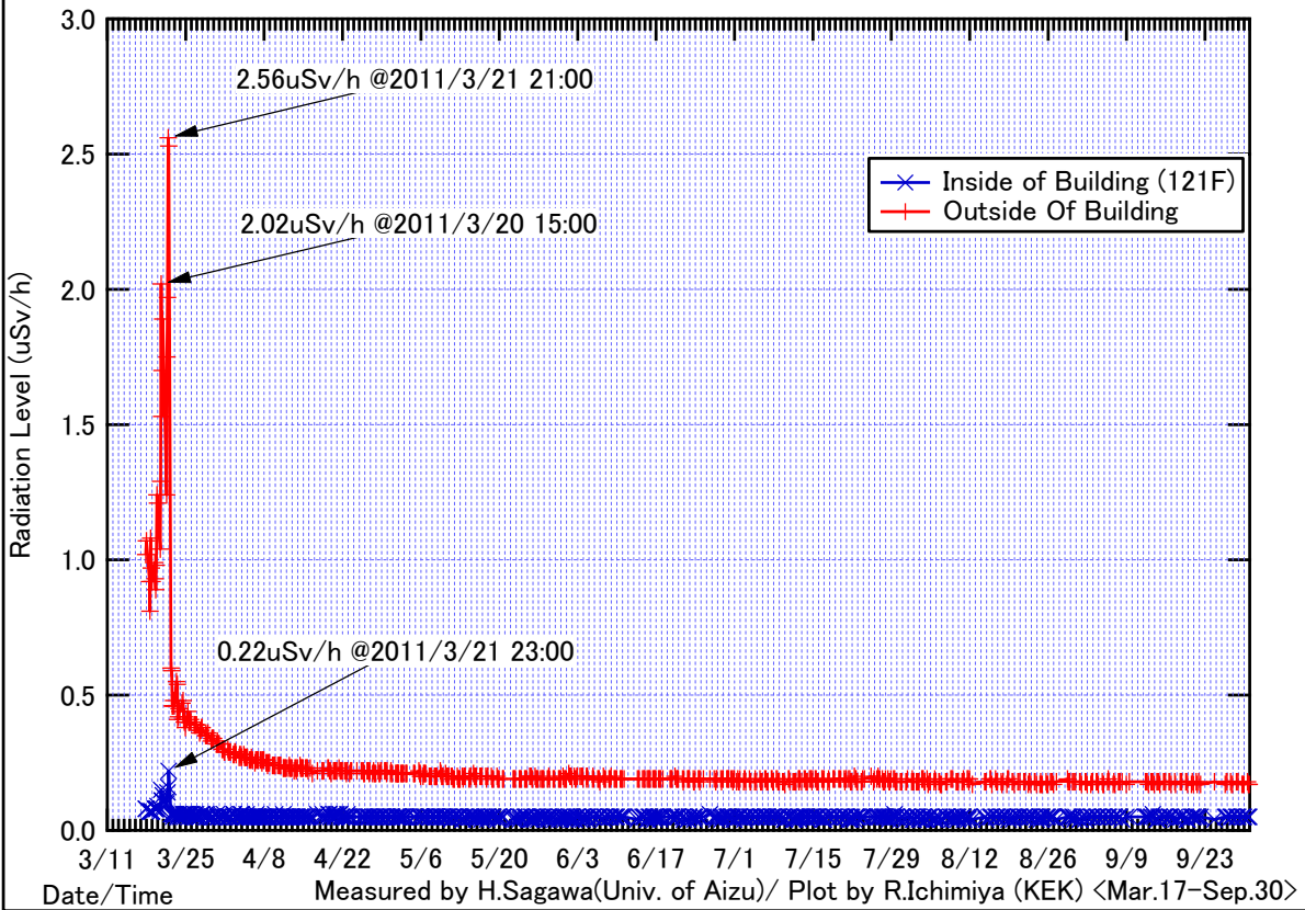
会津大学(福島県会津若松市)環境放射線レベル測定 (NaI) Environmental Radiation Level at Univ. of Aizu (Aizuwakamatsu, Fukushima)
